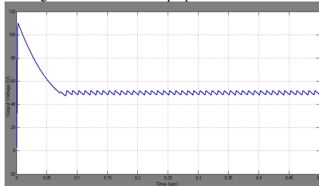
Fig. 9 Output Voltage
