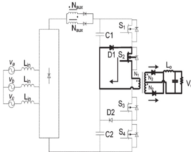
(c) Mode 3 ( t_2 < t < t_3 ).
