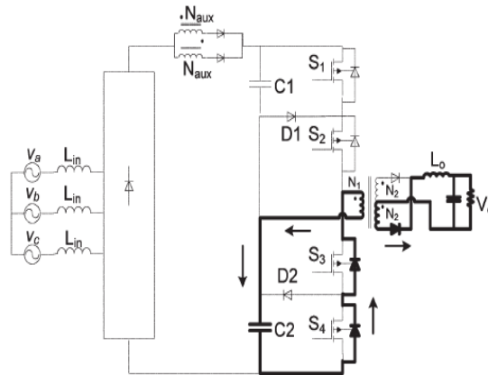
(d) Mode 4 ( t_3 < t < t_4 ). Fig. 4. Modes of operation
