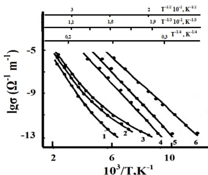
Fig. 4. Temperature dependences of electrical conductivity \sigma of composite polymer materials. The volume fraction of the filler in the composition 1 - 0.067; 2-0.080 and 3-0.088. 1-3 построены Графики в координатах \lg \sigma - 10^3/T . Данные для образца 2 представлены также в координатах \lg \sigma - T^{-1/4} (4), \lg \sigma - T^{-1/3} (5) и \lg \sigma - T^{-1/2} (6).
