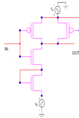
Fig. 12: 2PASCL inverter
