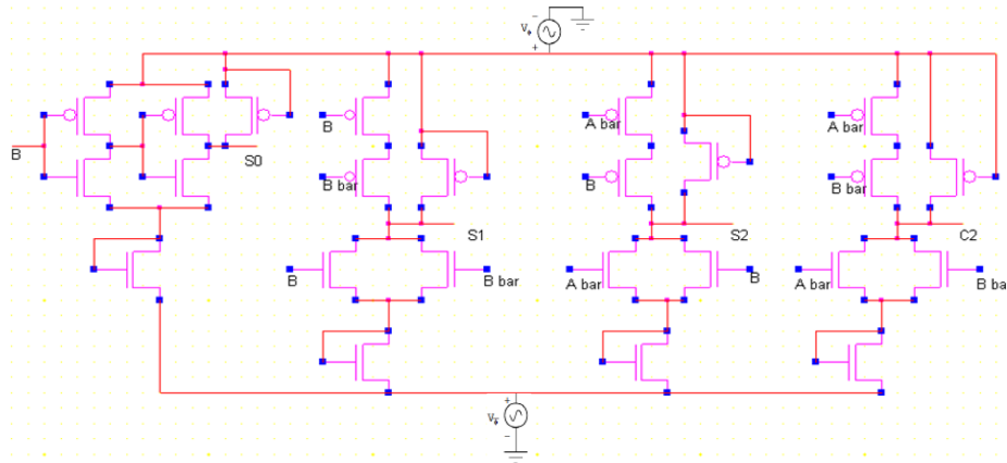
Fig. 13: 2PASCL Square
