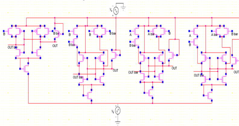
Fig. 15: PFAL & 2PASCL Square
