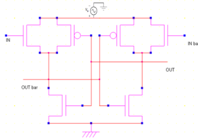
Fig. 10: PFAL inverter
