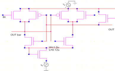
Fig. 14: PFAL&2PASCL inverter
